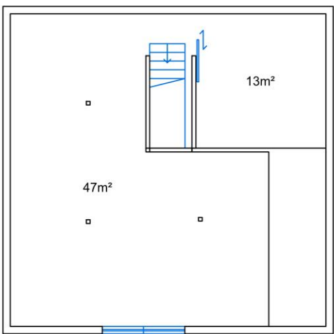
DACHGESCHOSS
